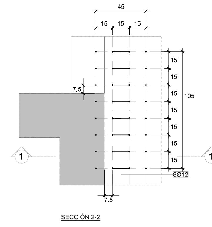
SECCIÓN 2-2
