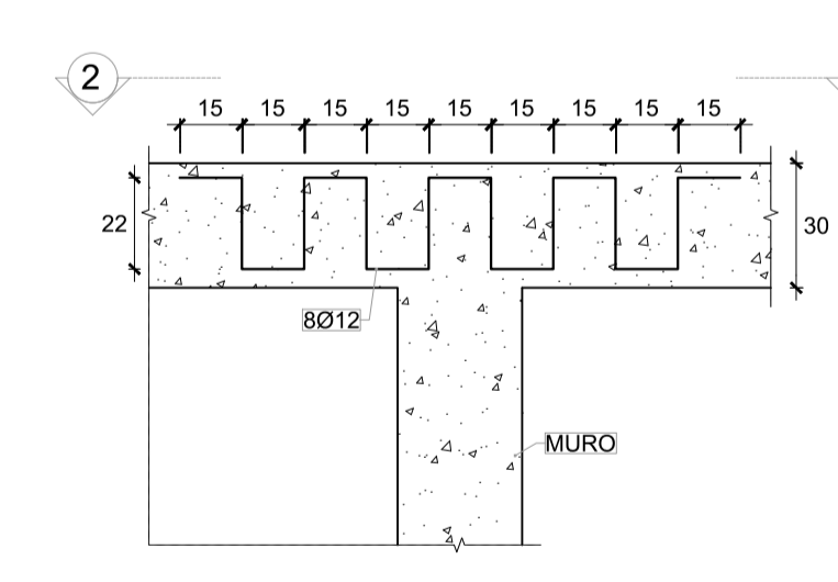
SECCIÓN 1-1
