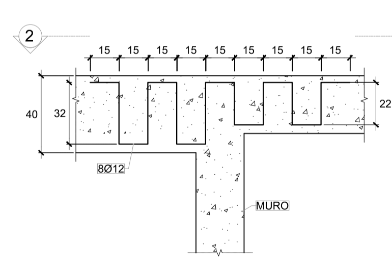
SECCIÓN 1-1
