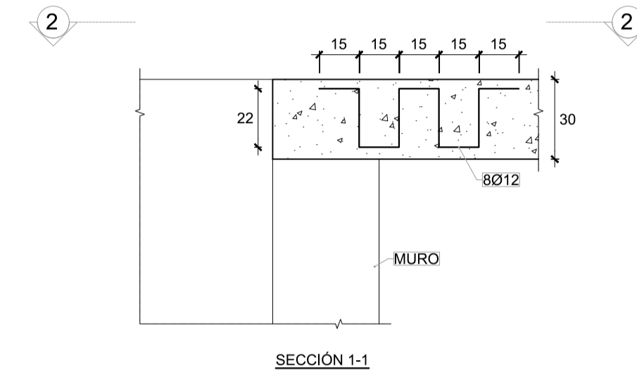
DETALLE DE ARMADO DE LOSA EN ENCUENTRO DE MUROS EJES H-2 EN NIVELES -2, -1 Y 0 ESCALA 1:20
