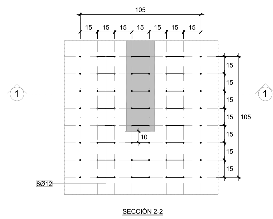
SECCIÓN 2-2
