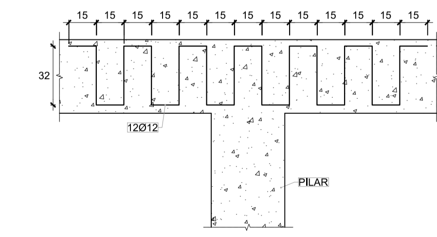
SECCIÓN 1-1
