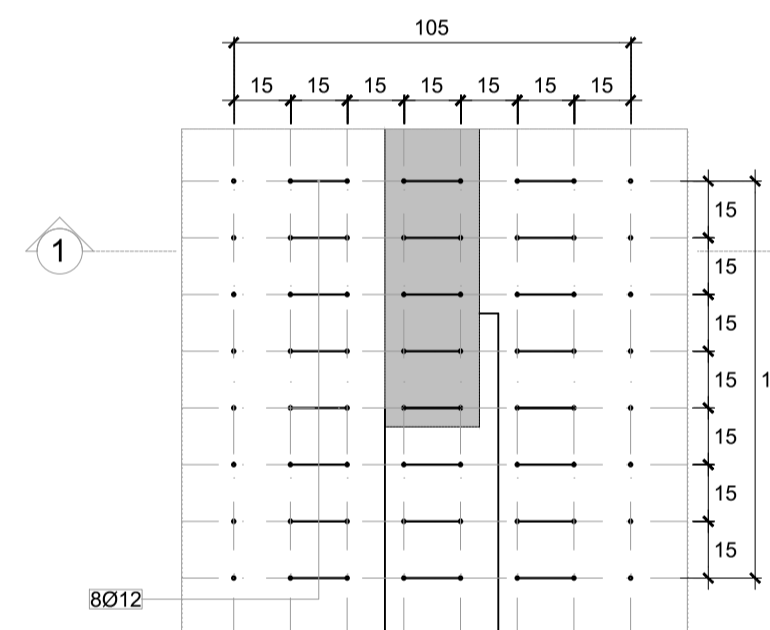
SECCIÓN 2-2
