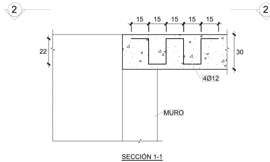
DETALLE DE ARMADO DE LOSA EN ENCUENTRO DE MUROS EJES B-18 Y K-6 EN NIVELES -2 Y -1 Y B-11 EN CUBIERTA ESCALA 1:20
