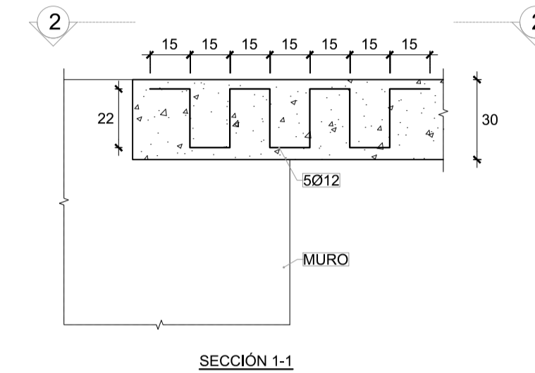
DETALLE DE ARMADO DE LOSA EN MURO EJE 18 EN NIVEL-2 ESCALA 1:20
