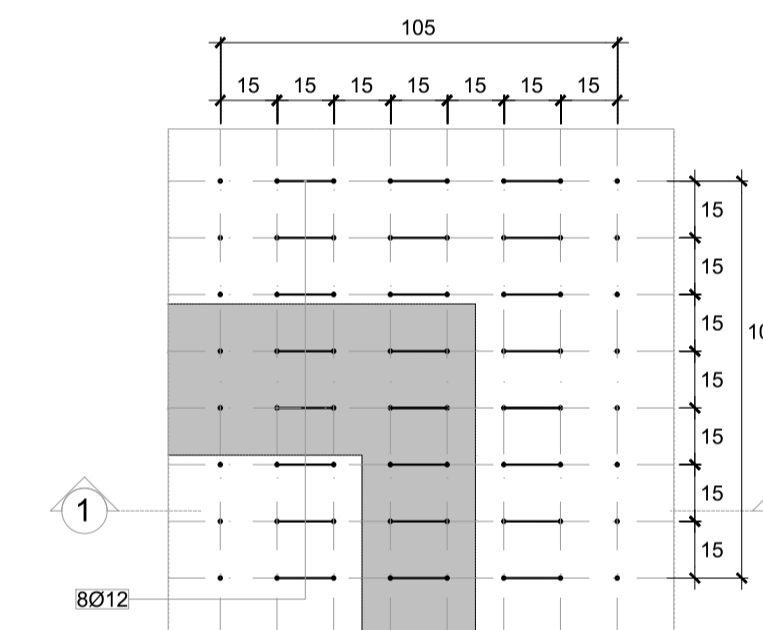
SECCIÓN 2-2
