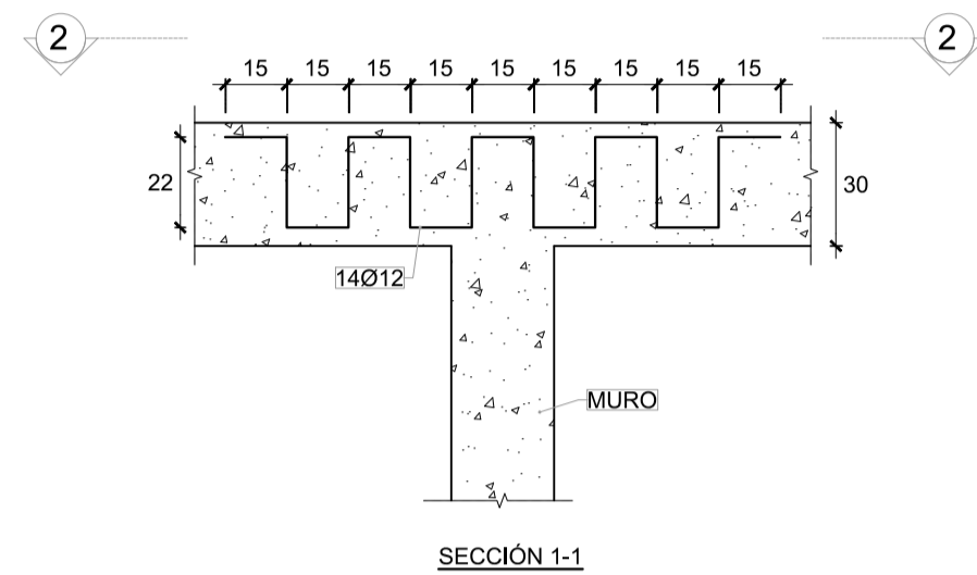
DETALLE DE ARMADO DE LOSA EN MURO EJE 10 EN NIVEL-2, TÉCNICA Y CUBIERTA, MURO EJE 8 EN NIVEL 2, 3 Y TÉCNICA, MURO EJE I EN NIVEL 3, Y MURO 14 EN CUBIERTA ESCALA 1:20
