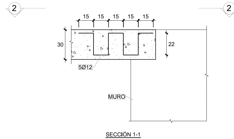
DETALLE DE ARMADO DE LOSA EN MURO EJE 14 EN NIVEL-2 ESCALA 1:20
