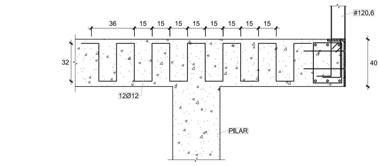
SECCIÓN 1-1
