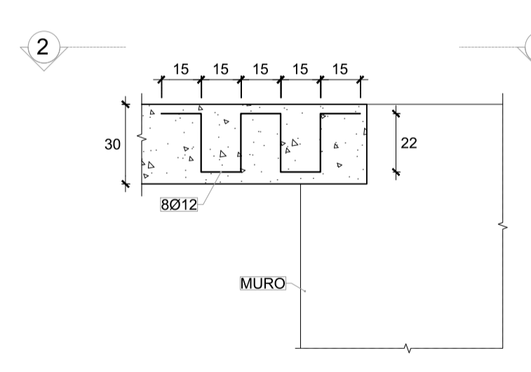
SECCIÓN 1-1
