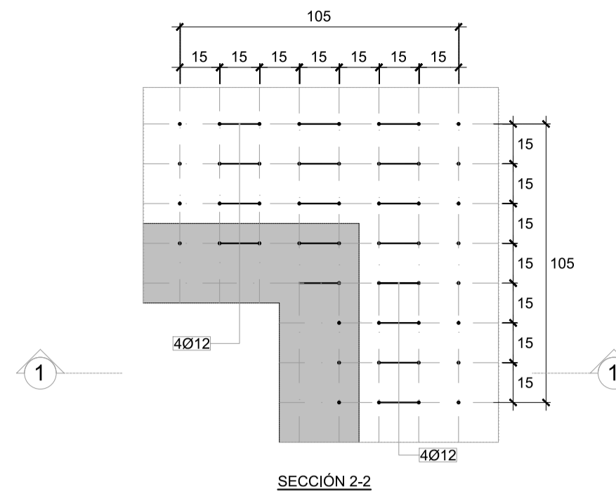
SECCIÓN 2-2
