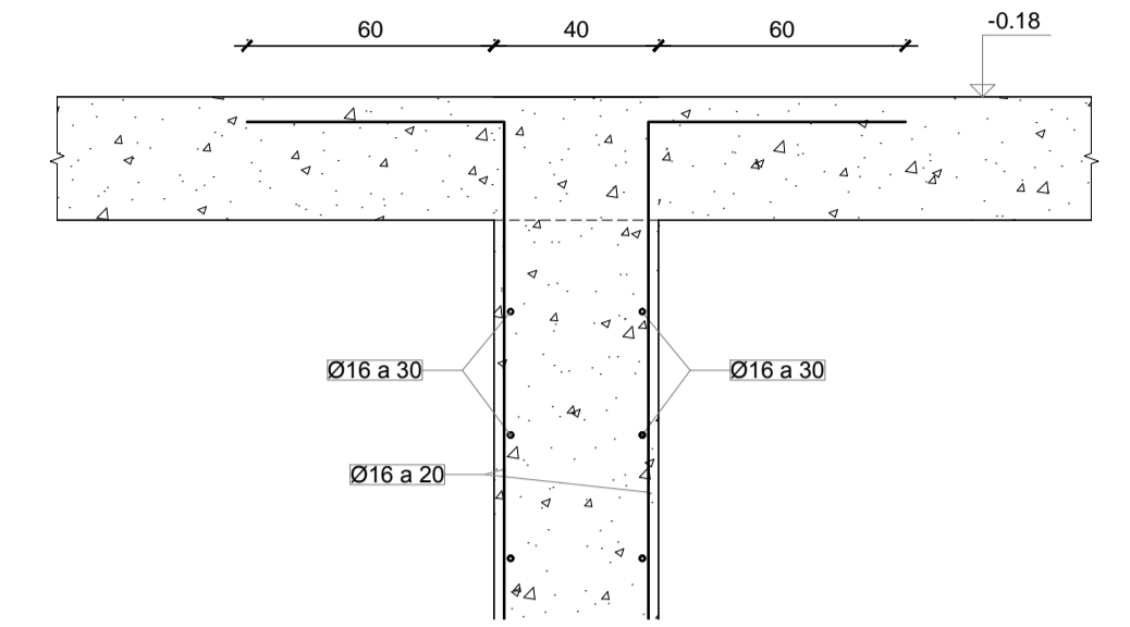
SECCIÓN CORONACIÓN MURO TIPO 11 BIS ESCALA 1:20
