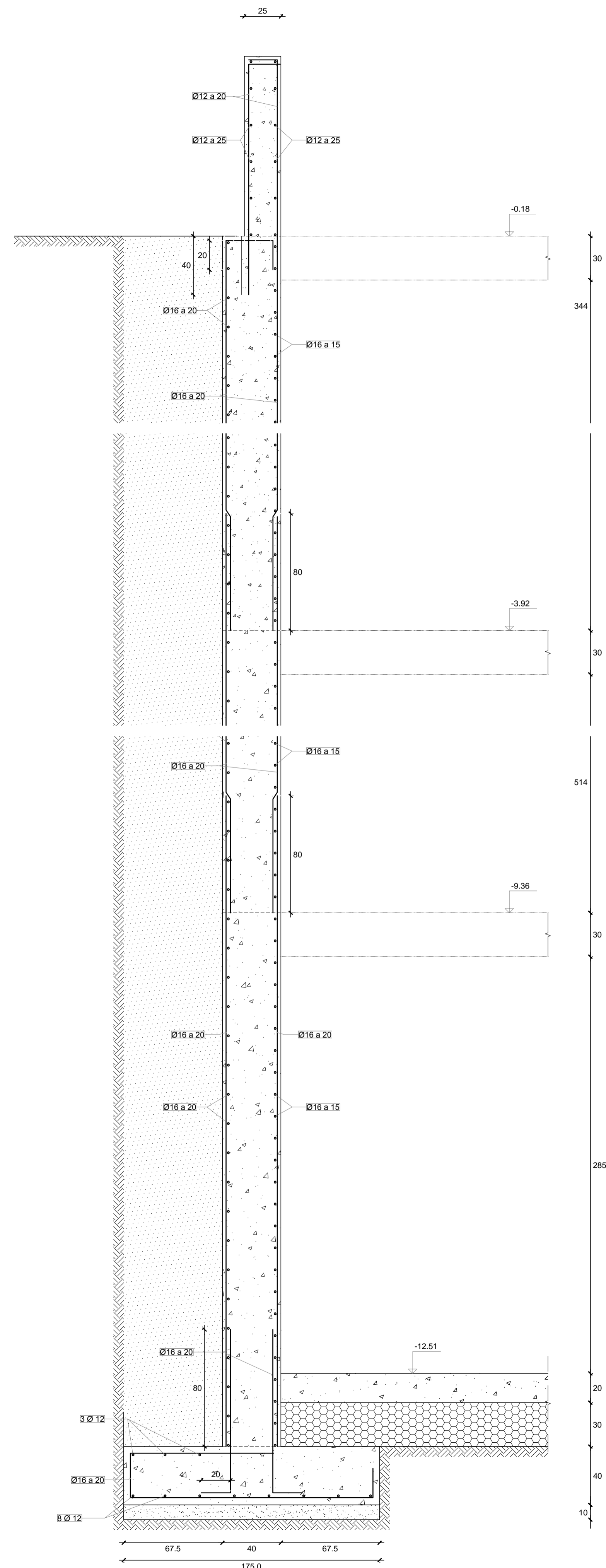
SECCIÓN MURO TIPO 10 ESCALA 1:20
