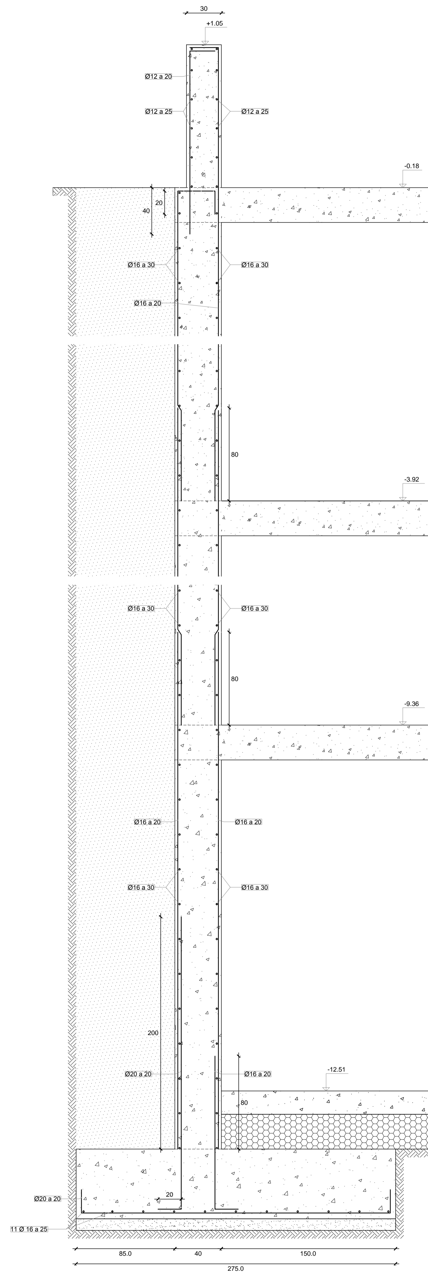
SECCIÓN MURO TIPO 11 ESCALA 1:20
