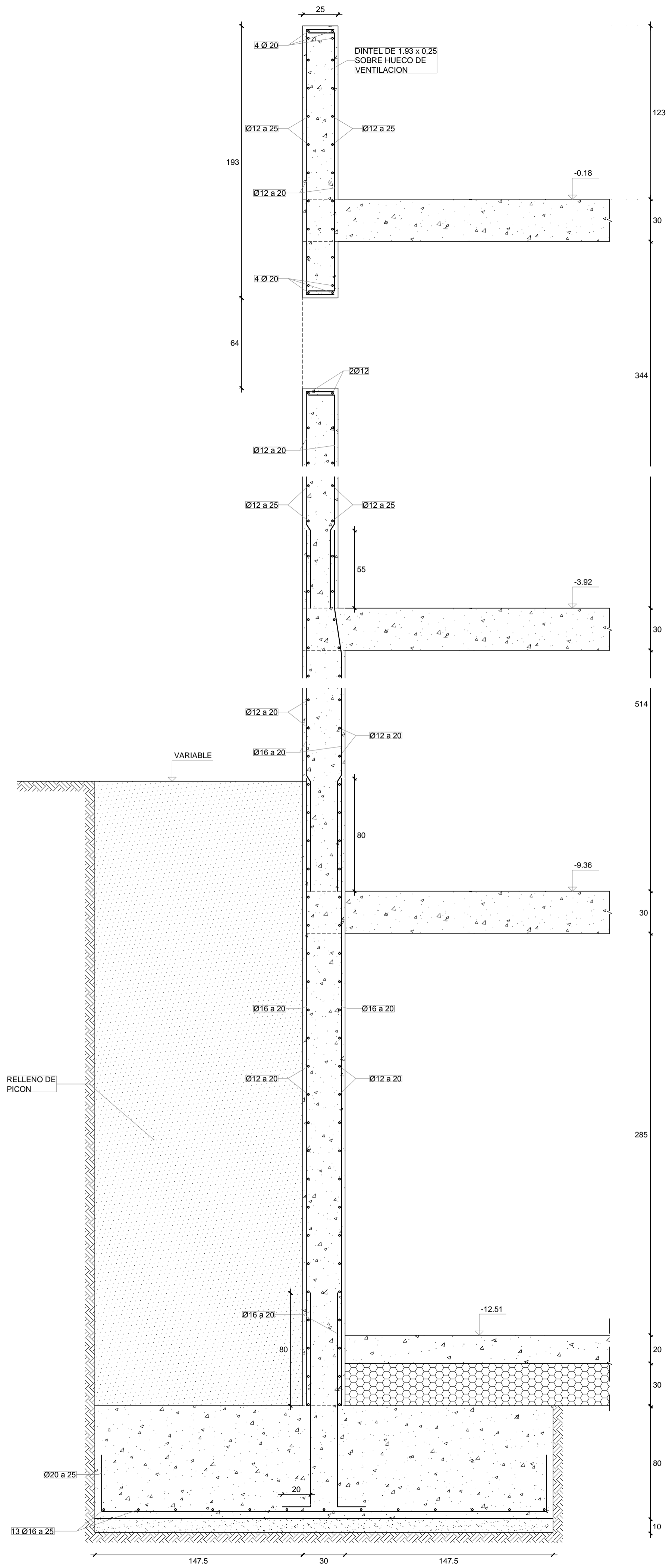
SECCIÓN MURO TIPO 7 ESCALA 1:20
