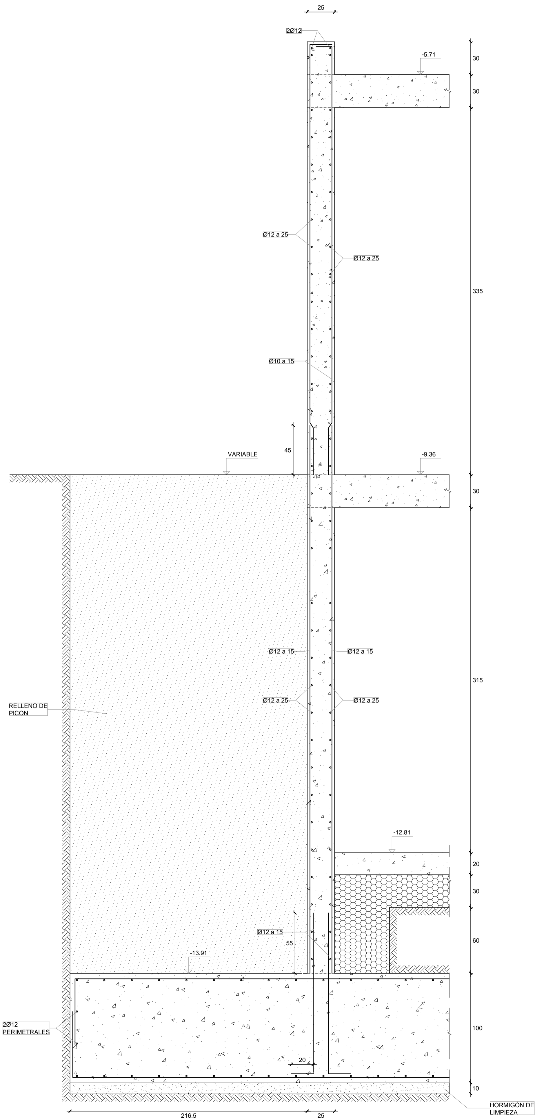
SECCIÓN MURO TIPO 6 BIS ESCALA 1:20
