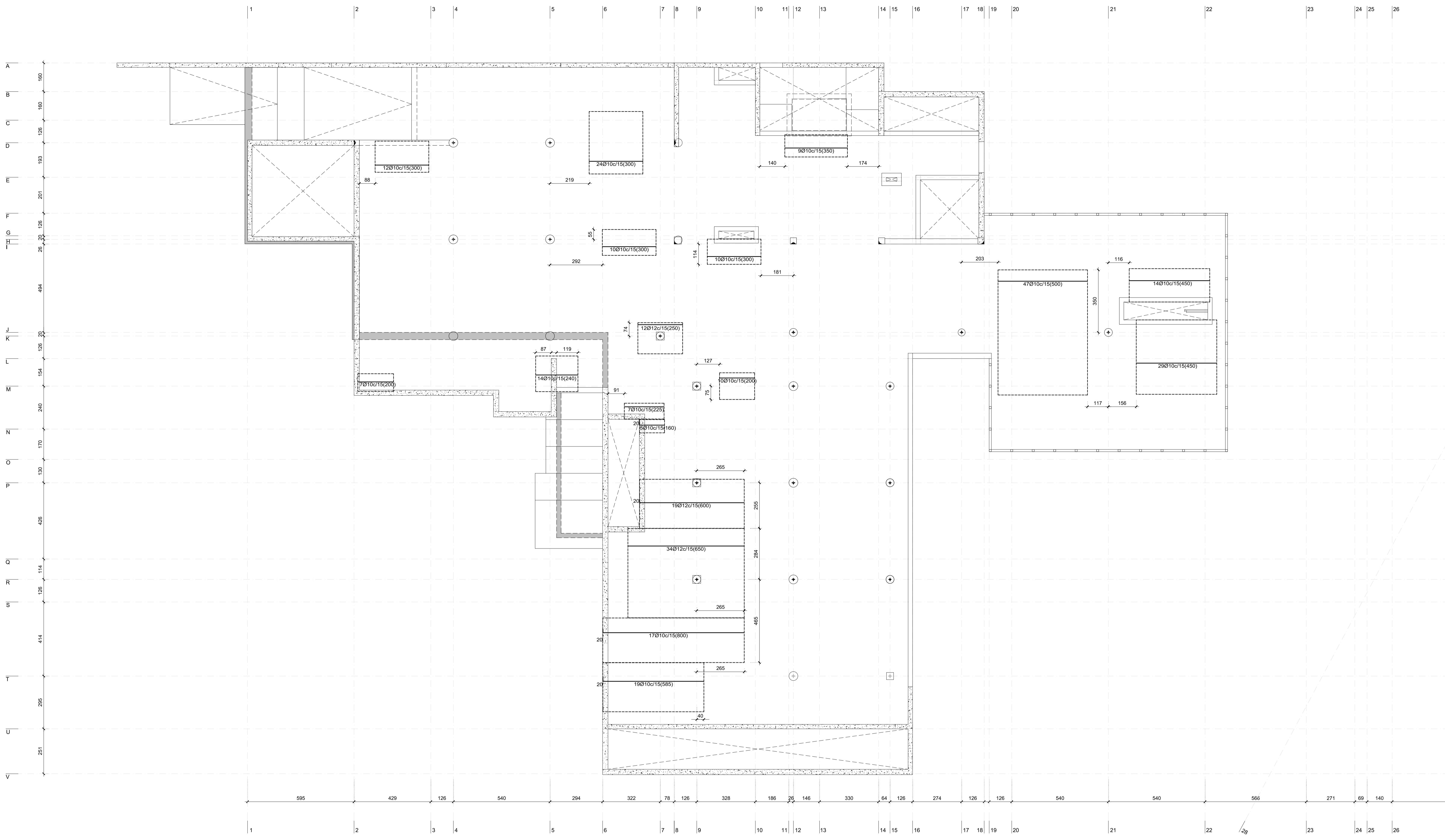
PLANTA NIVEL 0. (COTA -0.18 m) ESCALA 1:100
