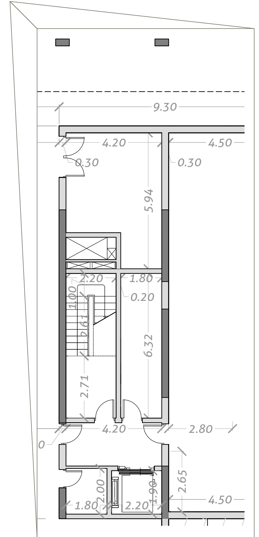
Núcleo de los módulos A, B y C E 1:100
